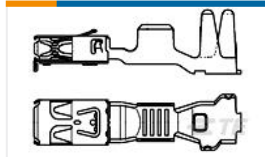
TE Part #1411594-1 ELOP2,8 F6000Y 65
