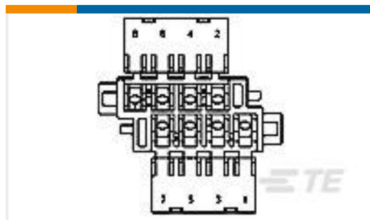
TE Part #365063-3 8P TAB HSG BLK
