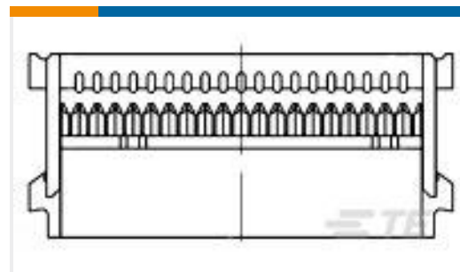
TE Part #1437021-5 609-2630=FSKT IDC S 26 30AU PL
