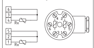
2x Dreileiterschaltung
