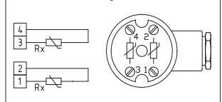
2x Zweileiterschaltung
