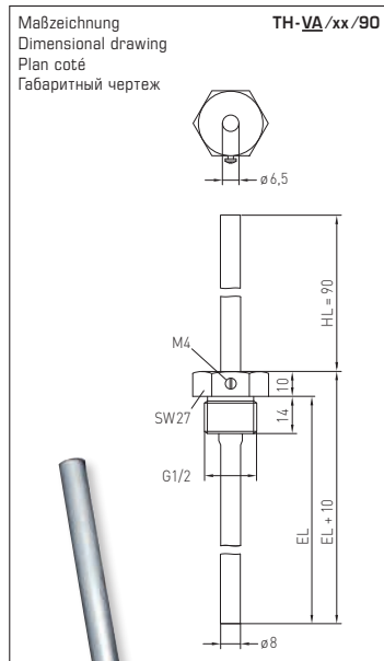
TH/xx/90 Edelstahltauchhülse mit Halsrohr Stainless steel immersion sleeve with neck tube doigt de gant en acier inox avec tube prolongateur Гильза погружная из высококачественной стали с горловиной
